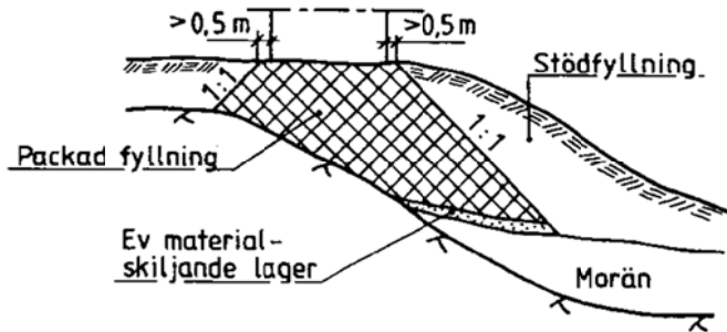
Figur E. 2 Minsta utsträckning av packad fyllning i plan och djup
