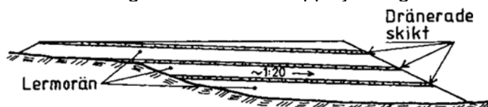
Figur E. 4 Vid packning av finkornig, vattenkänslig jord läggs skikten i lutning eventuellt med mellanliggande dränerande lager.
